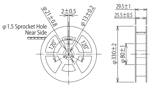
Reel Dimensions
